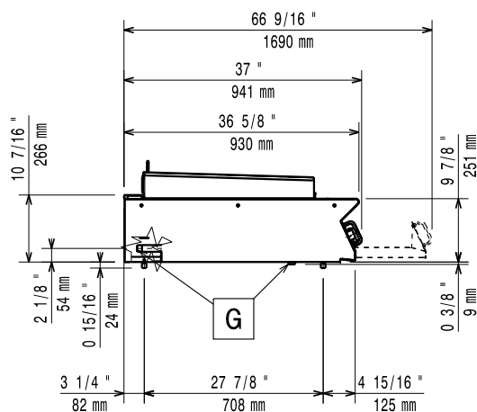
Zij aanzicht
